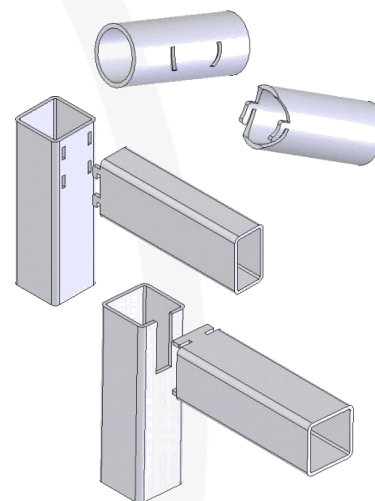
Haakverbindingen
